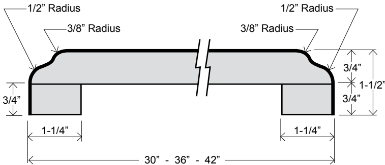
BAR TOP SVB 30 SVB 36 SVB 42
