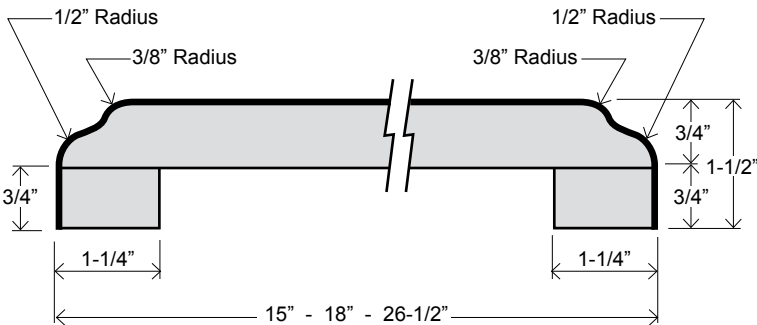
BAR TOP SVB 15 SVB 18 SVB 26-1/2
